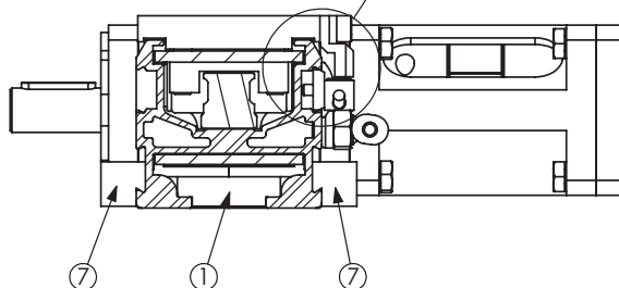
SEZIONE A-A
